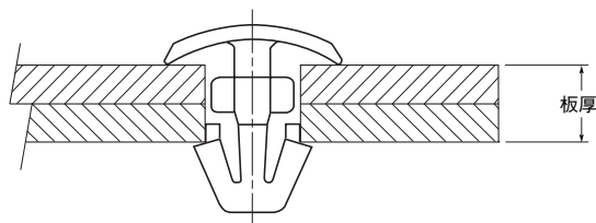
取付状態図
